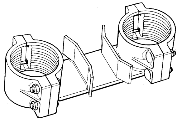
Guide central de barrière double poteau pour poteau 3-1/2 po Guide central de barrière double poteau pour poteau 4-1/2 po
