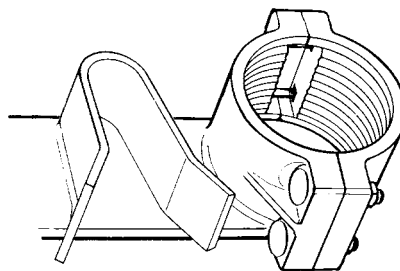
ARRÊT DE BARRIÈRE POTEAU UNIQUE DROIT OU GAUCHE — pour poteau 3-1/2 — pour poteau 4-1/2 po
