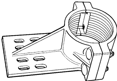
SUPPORTS DE RAIL POTEAU UNIQUE (Vis et écrous de rail non inclus) — pour poteau 3-1/2 — pour poteau 4-1/2 po
